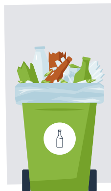
Vidro 5.359 kg
